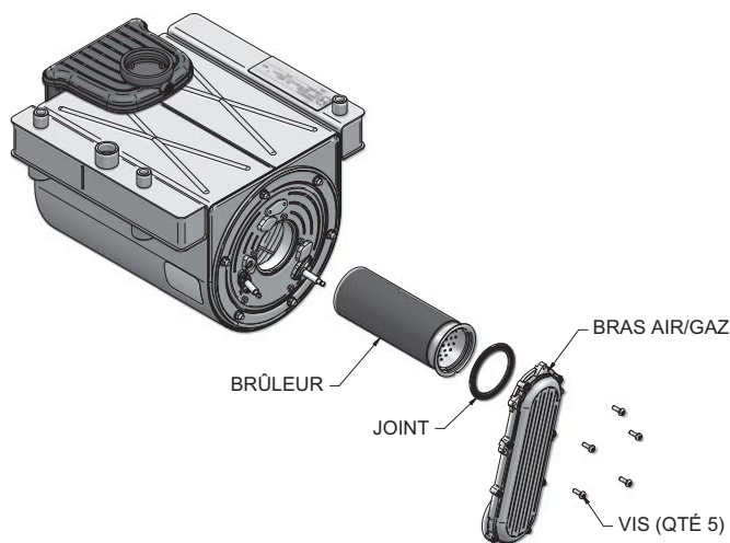
Figure 12-2 Ensemble brûleur
