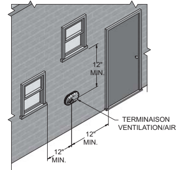
Figure 4-2B Espace alternatif par rapport aux entrées d'air gravitaires avec raccords fournis sur place
