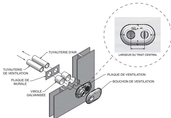
Figure 4-4A Ensemble de terminaison murale en PVC/CPVC
