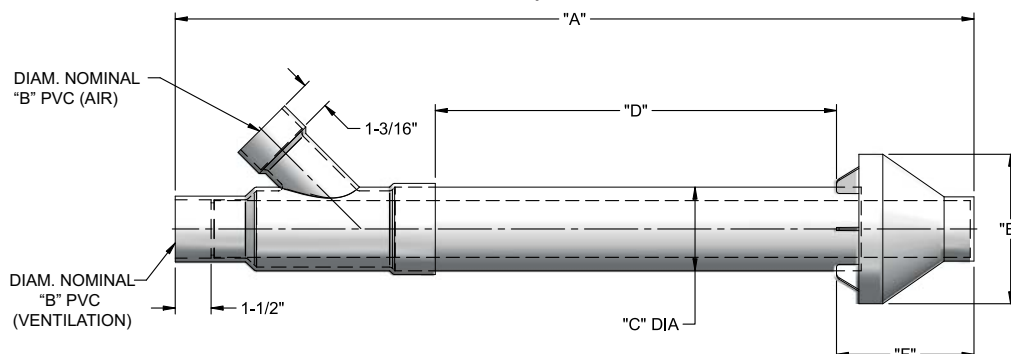
Figure 4-8 Schéma des dimensions de ventilation concentrique
