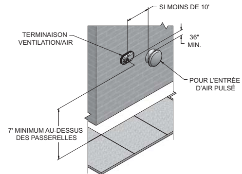
Figure 4-3A Espace par rapport aux entrées d'air forcé
