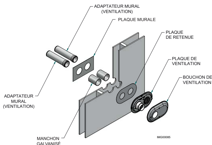
Figure 4-4B Ensemble de terminaison murale en polypropylène
