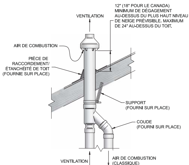
Figure 5-6 Installation de toit de ventilation concentrique
