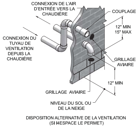
Figure 4-1D Disposition alternative de la ventilation – Terminaison latérale classique en acier inoxydable de la ventilation et de l'air avec raccords fournis sur place
