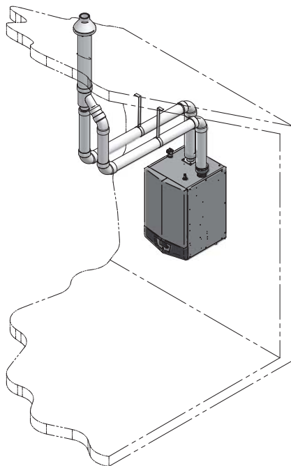
Figure 3-4 Terminaison verticale concentrique en PVC/CPVC - Voir page 31 pour d'autres détails
