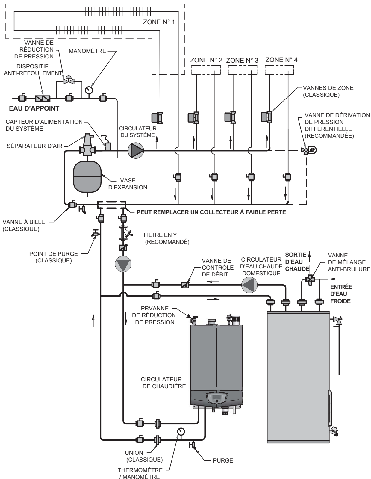
Figure 6-8 Chaudière unique Zonée avec vannes
