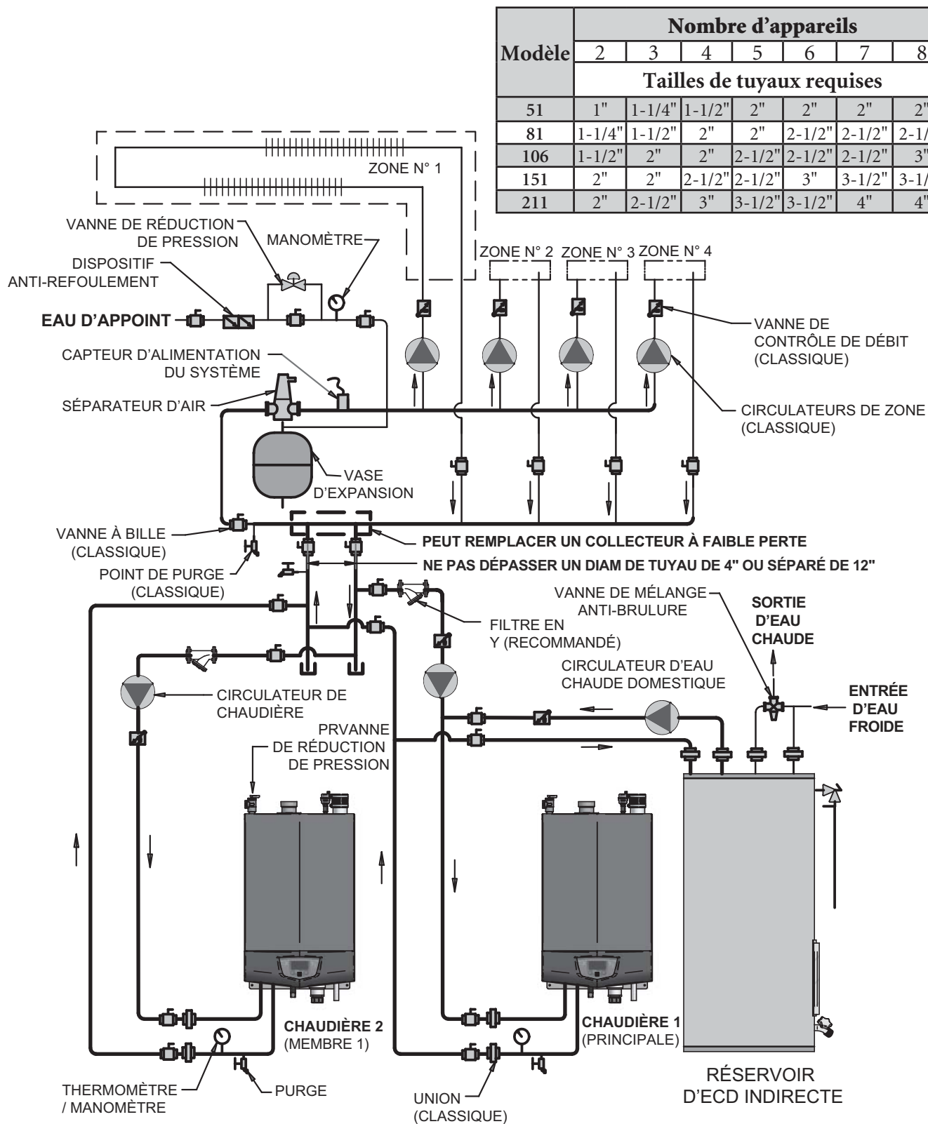
Figure 6-4 Chaudières multiples – Température unique zonée avec circulateurs
