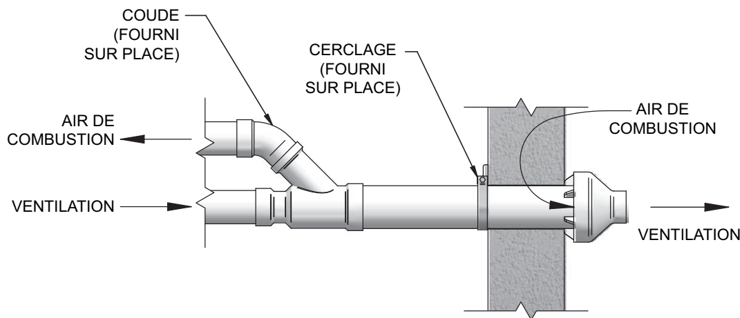
Figure 4-10 Fixation latérale de ventilation concentrique
