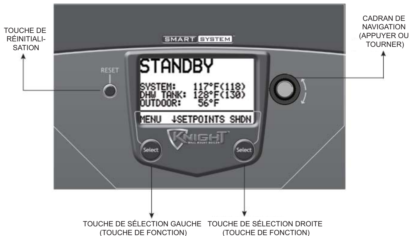
Figure 11-1 Panneau de commande
