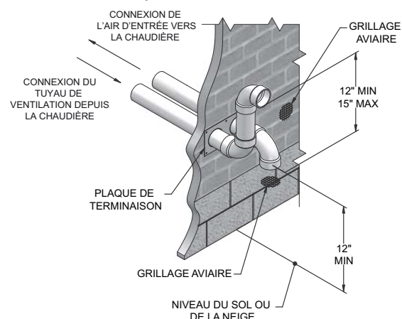
Figure 4-1B Terminaison latérale en PVC/CPVC/Polypropylène alternative d'air et de ventilation, avec raccords fournis sur place
