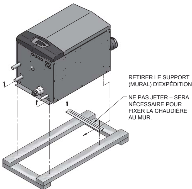
Figure 2-1 Chaudière montée sur une palette d'expédition
