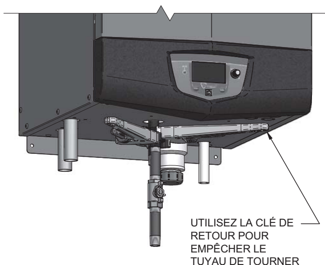
Figure 7-2 Tuyau d'entrée avec clé de retour
