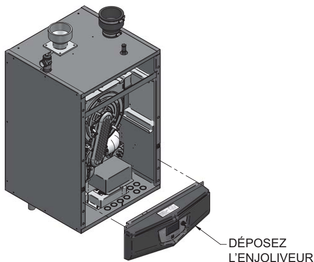
Figure 8-1 Dépose de l'enjoliveur
