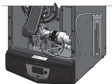
Figure 7-3 Vérification de l'alimentation en gaz d'entrée
