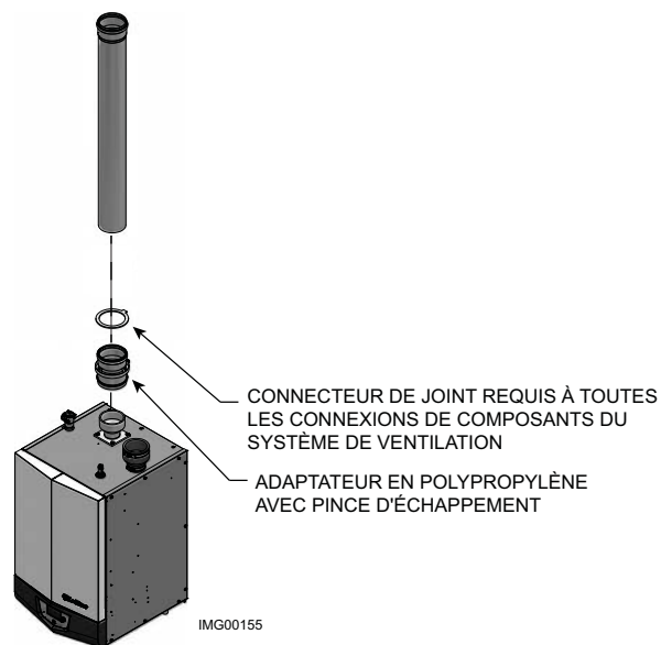
Figure 3-8 Ventilation en Polypropylène à proximité de la chaudière
