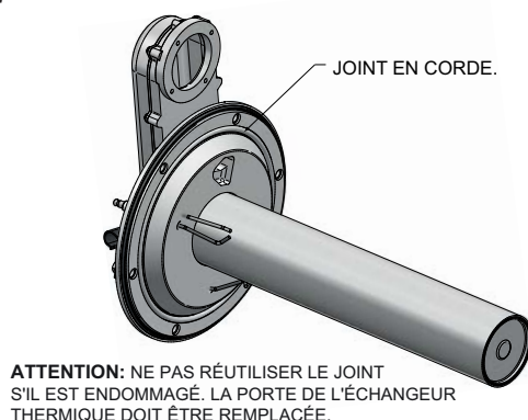
Figure 12-3 Joint en corde - Porte de l'échangeur thermique
