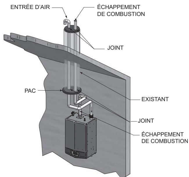
Figure 5-10 Ventilation existante en goutte
