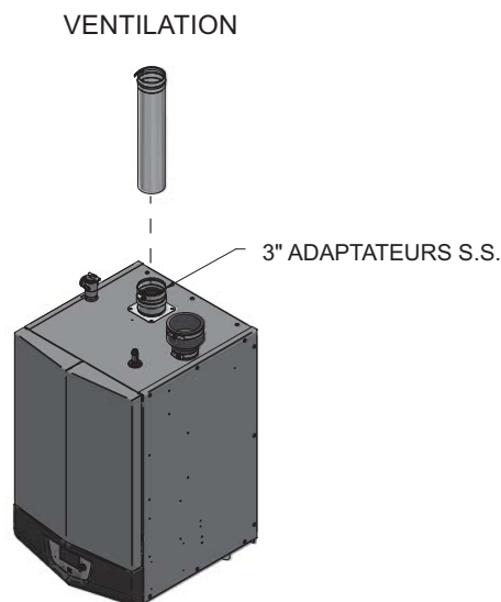
Figure 3-9 Près de la ventilation en acier inoxydable de la chaudière
