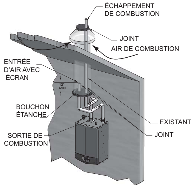
Figure 5-8 Exemple 1 de ventilation concentrique
