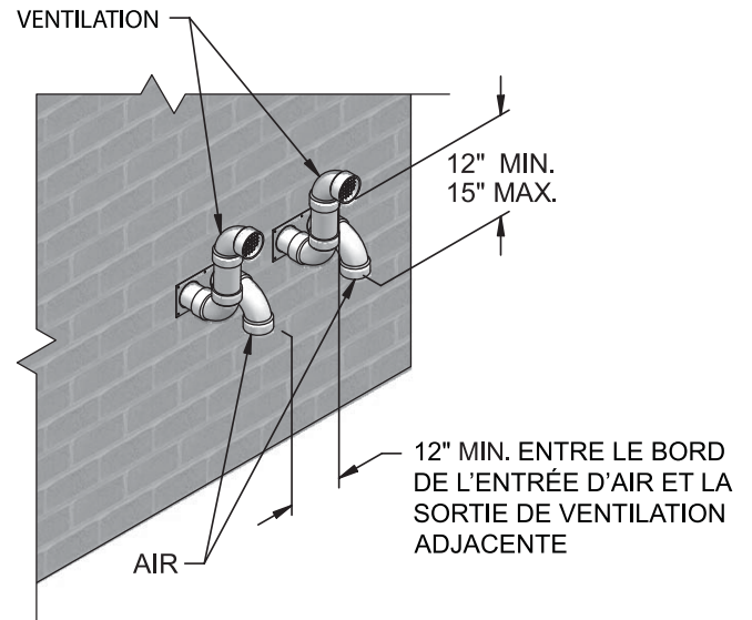
Figure 4-5B Terminaisons de ventilation multiple alternatives (doivent également être conformes à la Figure 4-1B )
