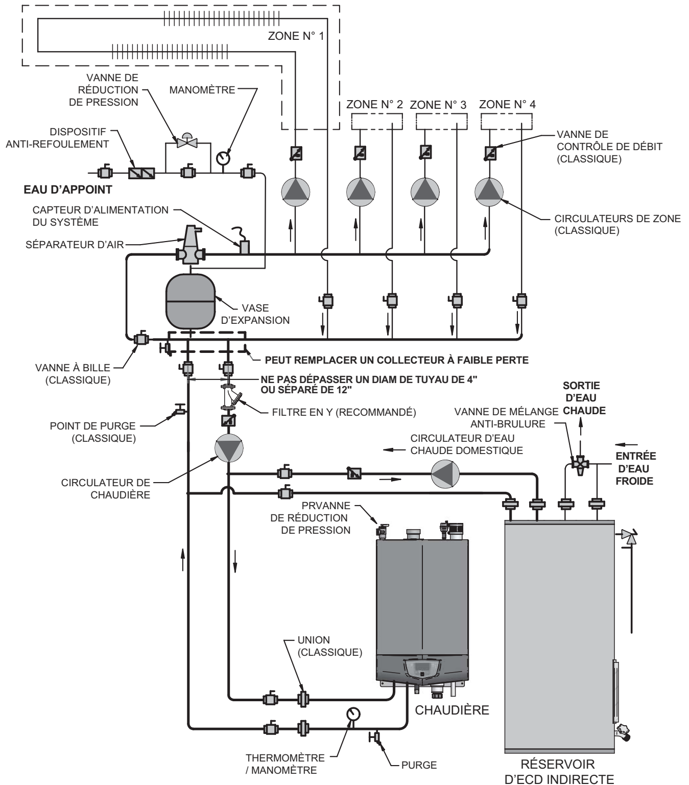
Figure 6-3 Chaudières unique – Température unique zonée avec circulateurs
