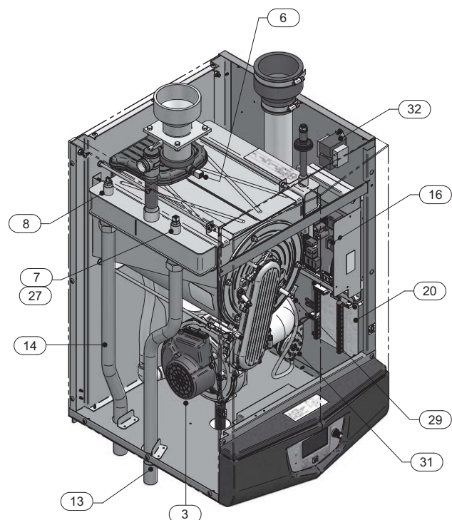
Vue de dessous (intérieur de l'appareil)
