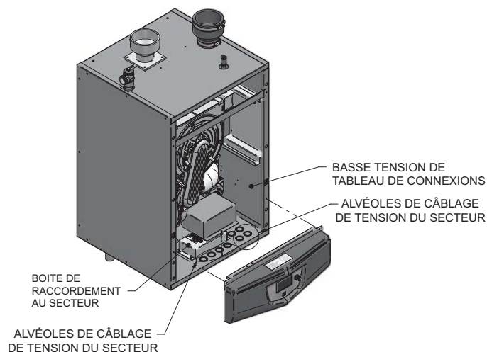
Figure 8-3 Acheminement des câbles sur place
