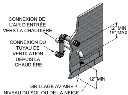
Figure 4-1D Disposition alternative de la ventilation – Terminaison latérale classique en acier inoxydable de la ventilation et de l'air avec raccords fournis sur place
