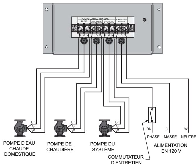
Figure 8-2 Connexions de câblage sur place au secteur
