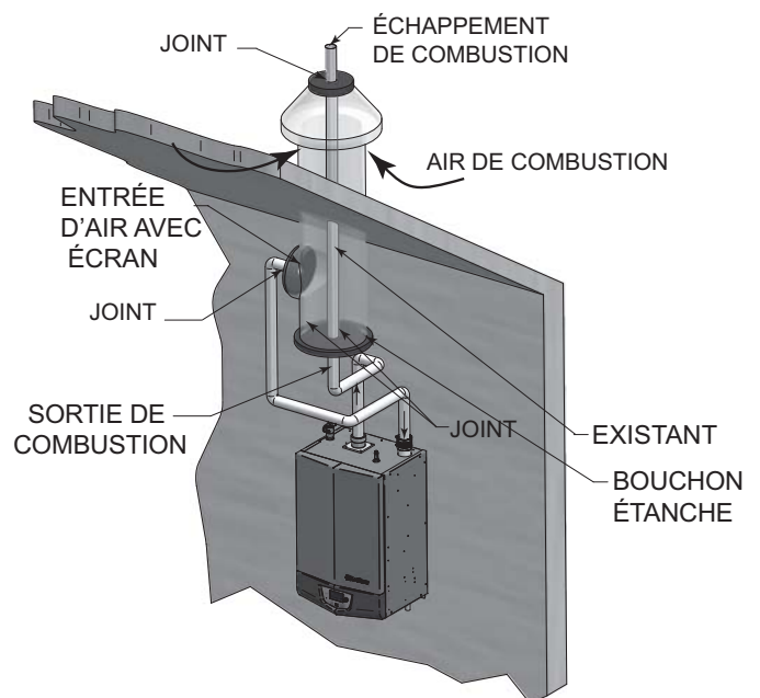
Figure 5-9 Exemple 2 de ventilation concentrique
